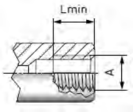
NPT螺纹(依据ANSI/ ASME B1.20.1-1983)
