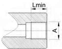
NPT-螺纹
