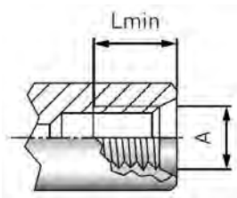
SAE螺纹(根据SAE J1926 / ISO 11926)
