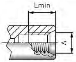
NPT螺纹 (ANSI/ ASME B1.20.1-1983)
