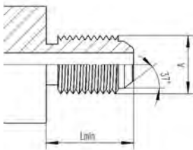
依据SAE J514 JIC37°标准
