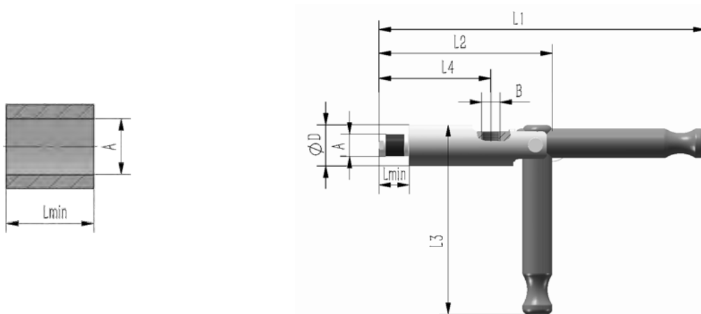
外形尺寸：1, 2, 3 型
