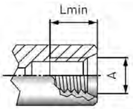
公制 ISO螺纹 (DIN 13 - 根据 ISO 6149-1)
