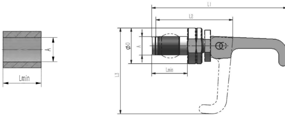
外形尺寸：1, 2, 3 型
